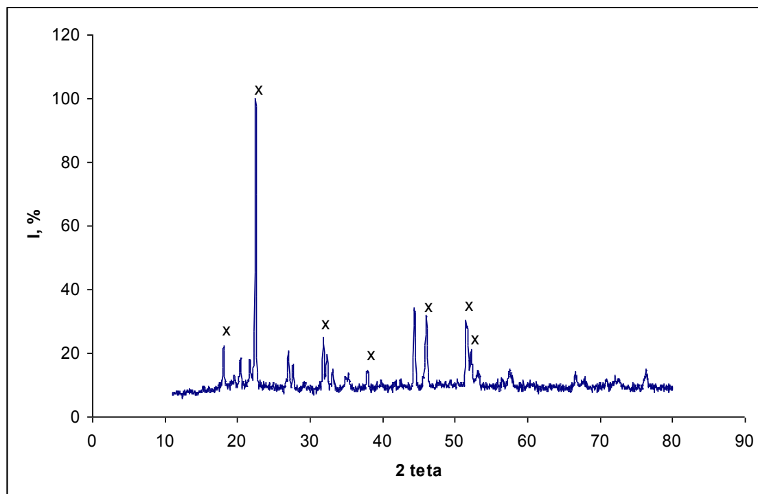
Рис.2. Рентгенограма охолодженого солявого сплаву з вихідним складом компонентів 54% \text{NiF}_2 – 46% \text{ZrF}_4
